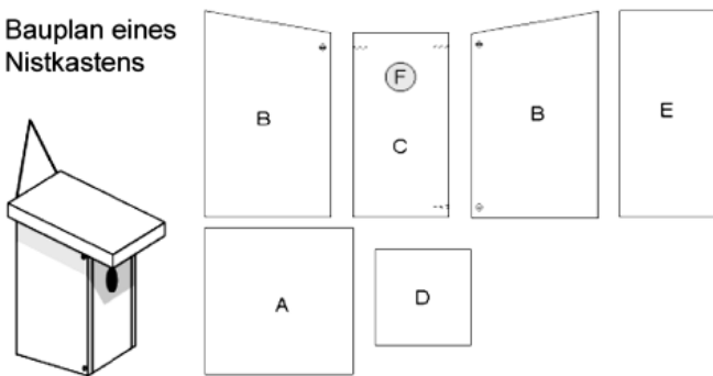
Maße eines Standardnistkastens mit quadratischer Grundfläche (cm)
